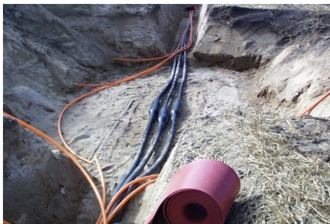
Figur 2-43 Kablerne er muffet sammen
