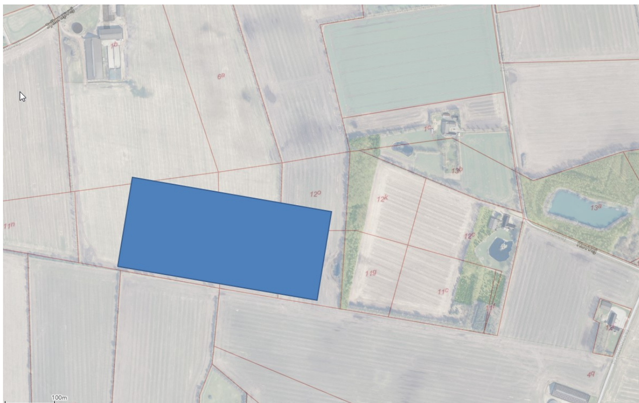
Figur 4-4. Den nye koblingsstation placeres i Varde Kommune nord for den eksisterende station Endrup og tilkøbes denne. Arealet til stationen udgør ca. 7,2 ha (400x180m).
