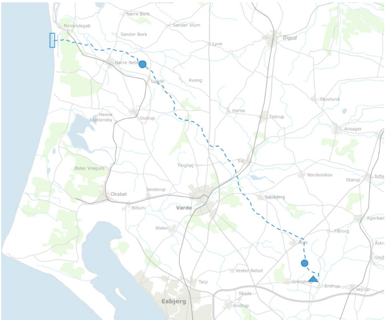
Figur 1-1 Placering af projektet Mere Havvind 2030 Nordsøen I-A2 til Endrup, hvor firkanten angiver placering af ilandføringspunktet, cirklerne angiver placering af koncessionvinders anlæg (nord: kompensationsstation, syd: koblingsstation) og trekanten angiver placering af eksisterende højspændingsstation ved Endrup. Den stiplede linje angiver placering af landkabeltracé.
