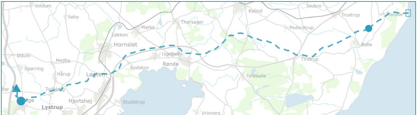
Figur 1-2 Placering af projektet Mere Havvind 2030 Kattegat Havvindmøllepark til Trige, hvor firkanten angiver placering af ilandføringspunktet, cirklerne angiver placering af koncessionsvindens anlæg (øst: kompenseringsstation, vest: koblingsstation) og trekanten angiver placering af eksisterende højspændingsstation ved Trige. Den stiplede linje angiver placering af landkabeltracé.
