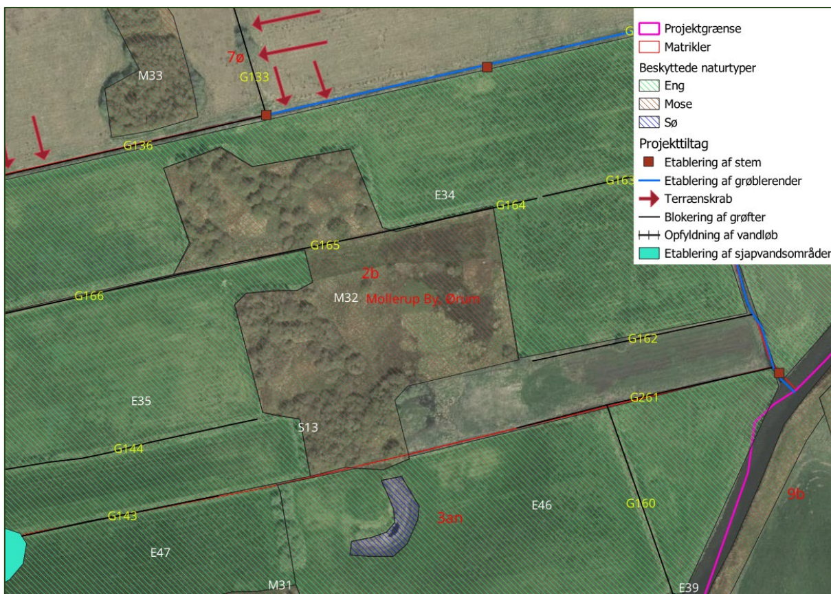
Figur 119. Projekttiltag i og omkring mose M32.
