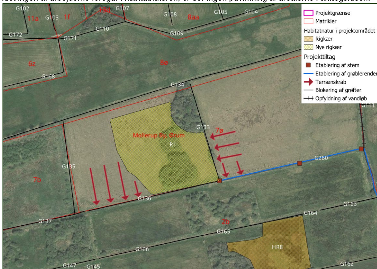
Figur 76. Projekttiltag i og omkring det nye riggær R1.
