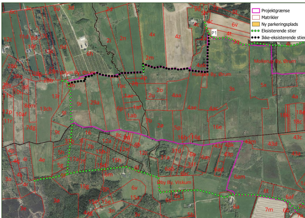
Figur 41. Placering af parkeringsplads samt sti mod Møllerup og til Ørum via Søndermarksvej og til Ø Bakker. Nye stiforløb uden for projektområdet etableres
