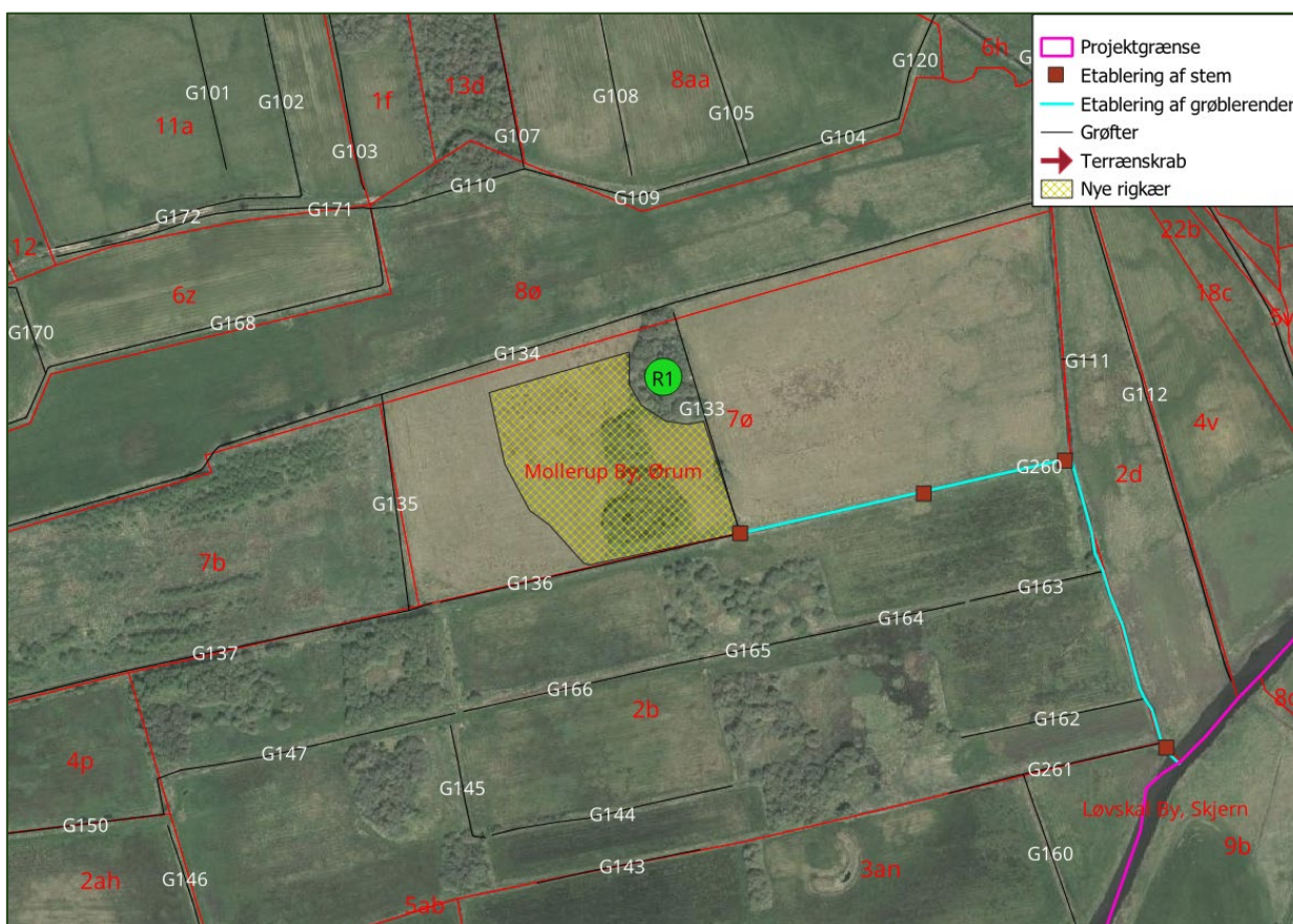
Figur 18: Lokaliseret rigkær (R1) på 1,5 ha. på matr. nr. 7ø Mollerup By, Ørum med tiltag, der skal sikre fortsat vandgennemstrømning igennem rigkæret efter en projekterisering. De hvide numre angiver grøfter i området.
