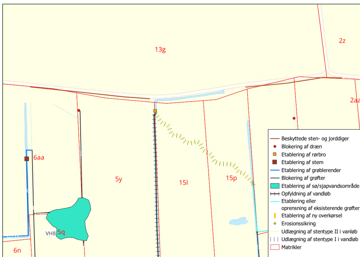
Figur 43: Projekttiltag ved tre beskyttede jord- og stendiger (mørkebrun streg).
