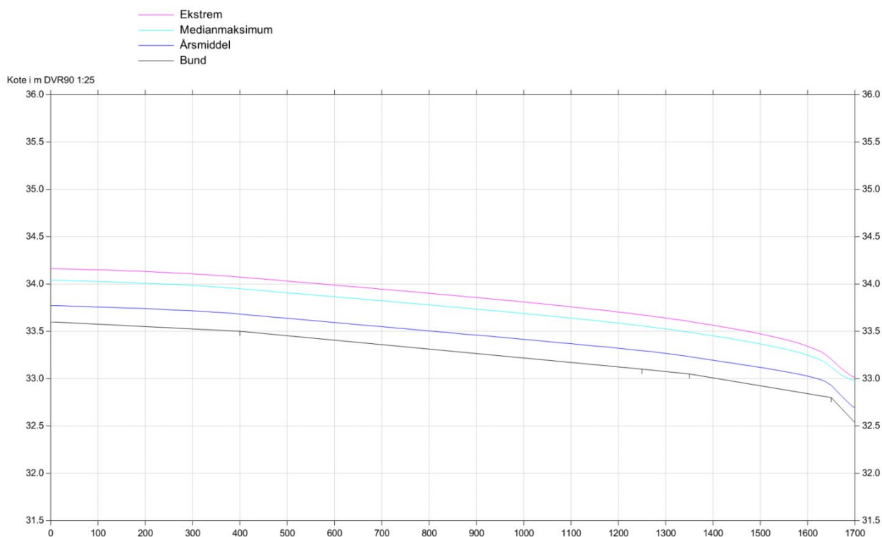
Figur 4-1 Beregnede vandspejle
