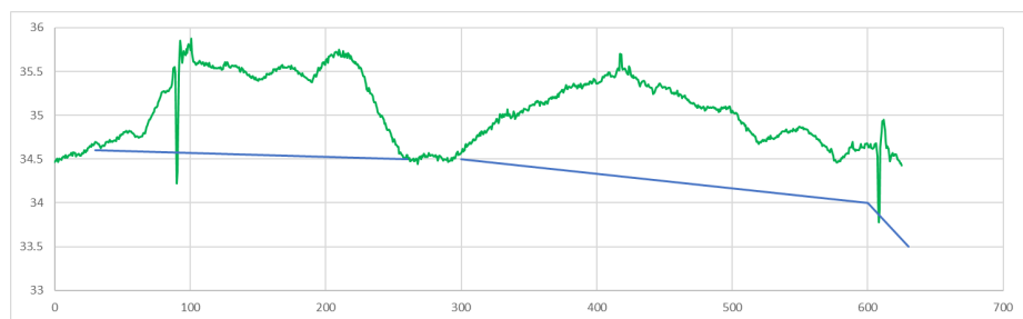
Figur 3-4 Længdesnit af terræn langs Tilløb fra øst. Lavning A er ved st. 0-30 og lavning B ved st. 260-300.
