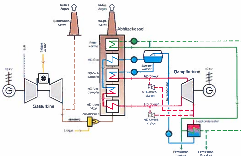
Illustration 3-1: Skematisk fremstilling af GuD-anlægget (Kedel 13)
