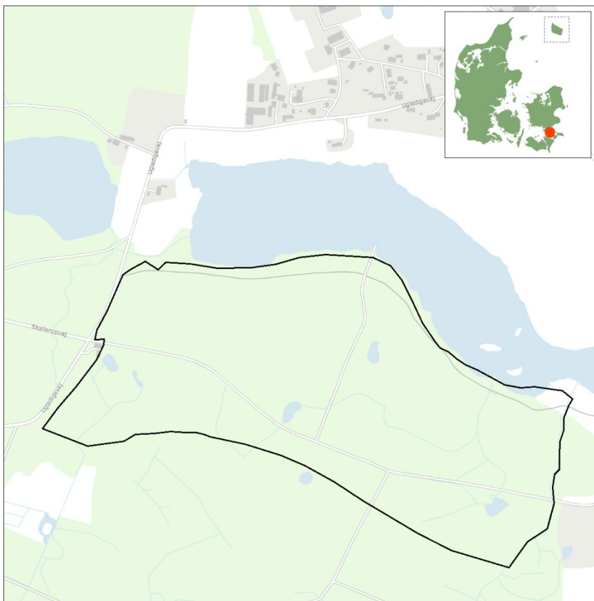
Figur 1. Gældende afgrænsning af Natura 2000-området N172 Lekkende Dyrehave.
