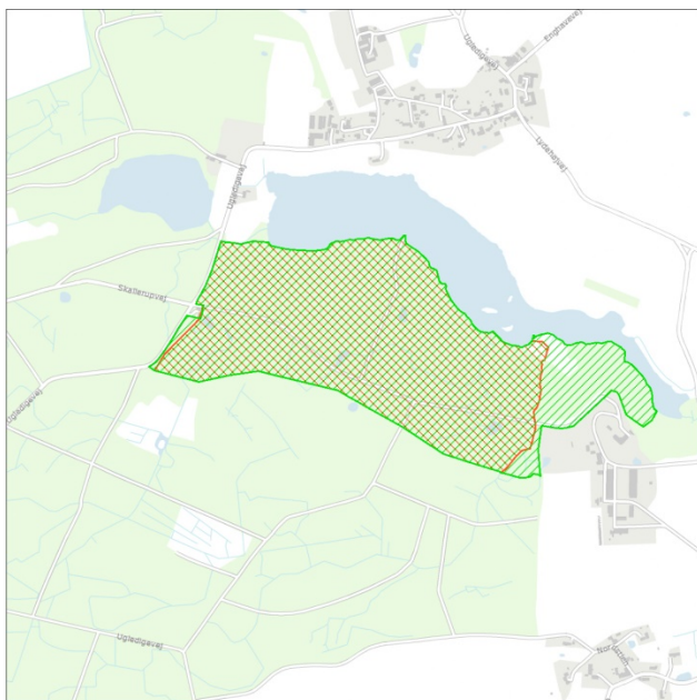
Figur 3. Habitatområde H151 Lekkende Dyrehave. Den røde skravering viser de berigtigede grænser for habitatområdet, og den grønne skravering angiver høringsforslagets afgrænsning. Dvs. at arealer, der kun er skraveret med grønt, er arealer, der er foreslået tilføjet til det beskyttede område.
