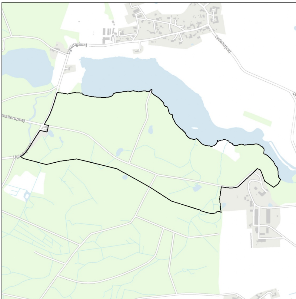
Figur 4. Den endelige afgrænsning af Natura 2000-område N162 Skælskør fjord og havet og kysten mellem Agersø og Glænø fremgår af kortet.
