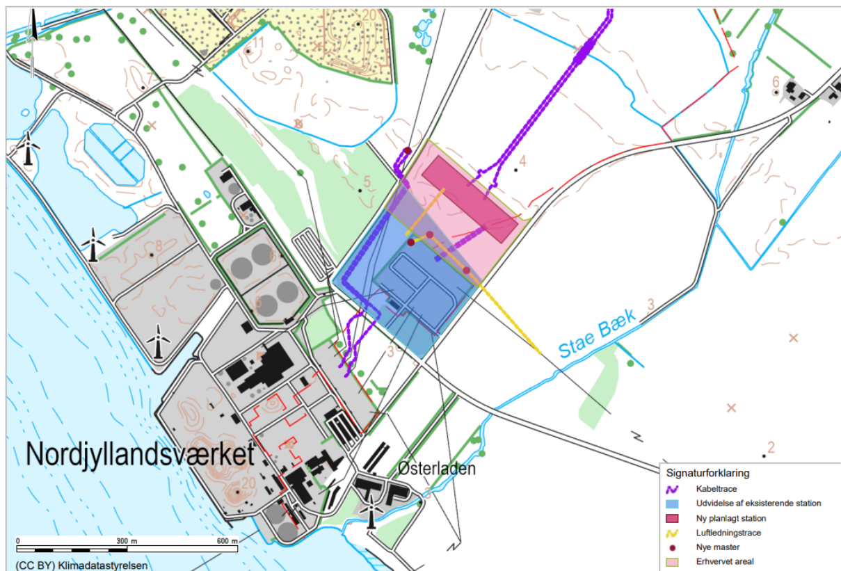
Figur 1-3 Placering af ny 150 kV højspændingsstation, Vendsysselværket, samt markering af det areal, som Energinet erhverver til vandhåndtering mv. omkring den nye station. Desuden udvidelse af den eksisterende 400 kV højspændingsstation, 400 kV Vendsysselværket. Herudover er markeret nye jordkabler samt etablering af ny luftledning og opsætning af enkelte master. Se evt. kortet fra Energinets hjemmeside: Indpasning af VE i Nordjylland - Vest
