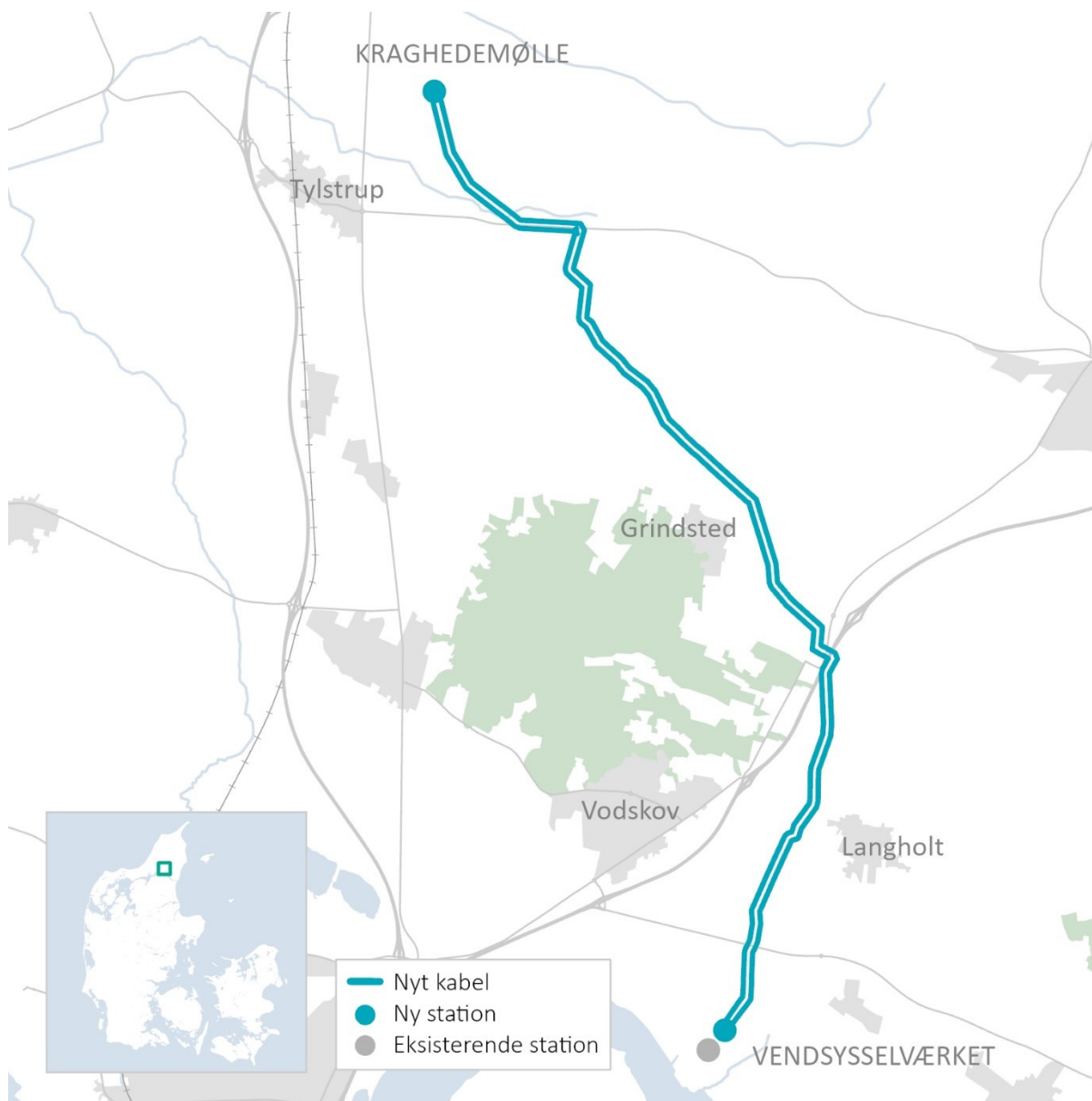
Figur 1-1. Placering af projektet med markering af de to nye 150 kV højspændingsstationer Kraghedemølle og Vendsysselværket, den eksisterende højspændingsstation 400 kV Vendsysselværket, der udvides, samt jordkablerne, der forbinder stationerne.
