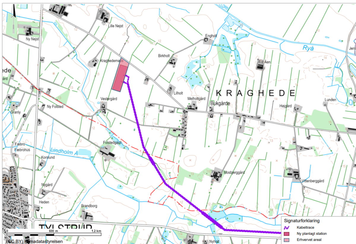
Figur 1-2 Placering af ny 150 kV højspændingsstation, Kraghedemølle, samt markering af det samlede areal, som Energinet erhverver til vandhåndtering mv. Se evt. kortet fra Energinets hjemmeside: Indpassning af VE i Nordjylland - Vest
