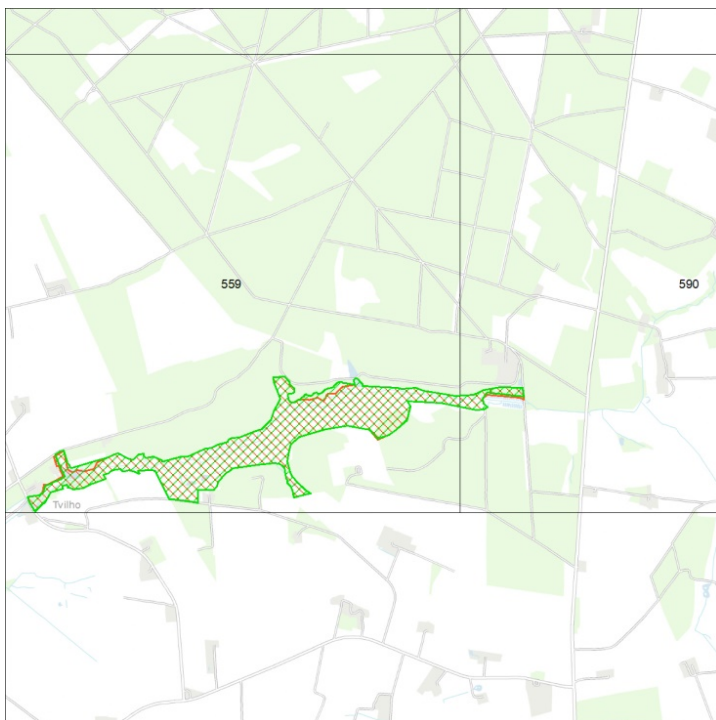
Figur 4. Habitatområde H76 Nørrebæk ved Tvilho. Den røde skravering viser de berigtigede grænser for habitatområdet, og den grønne skravering angiver høringsforslagets afgrænsning.
