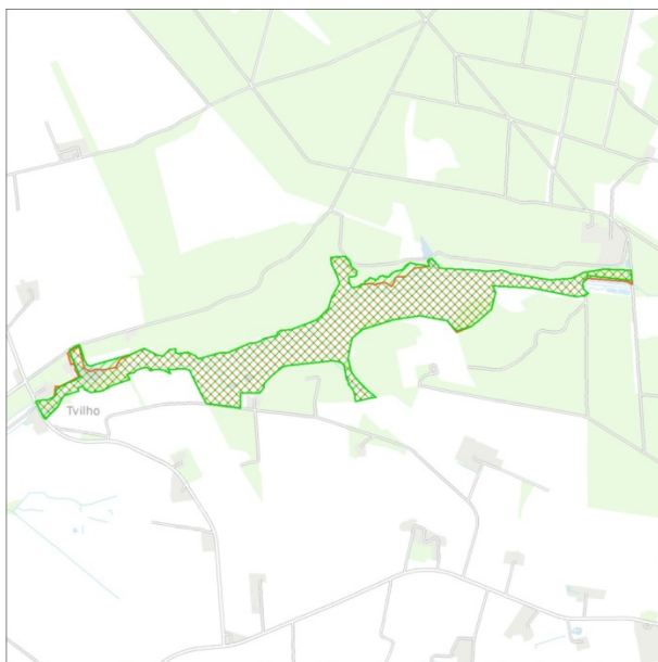
Figur 3. Habitatområde H76 . Den røde skravering viser de berigtigede grænser for habitatområdet, og den grønne skravering angiver høringsforslagets afgrænsning.
