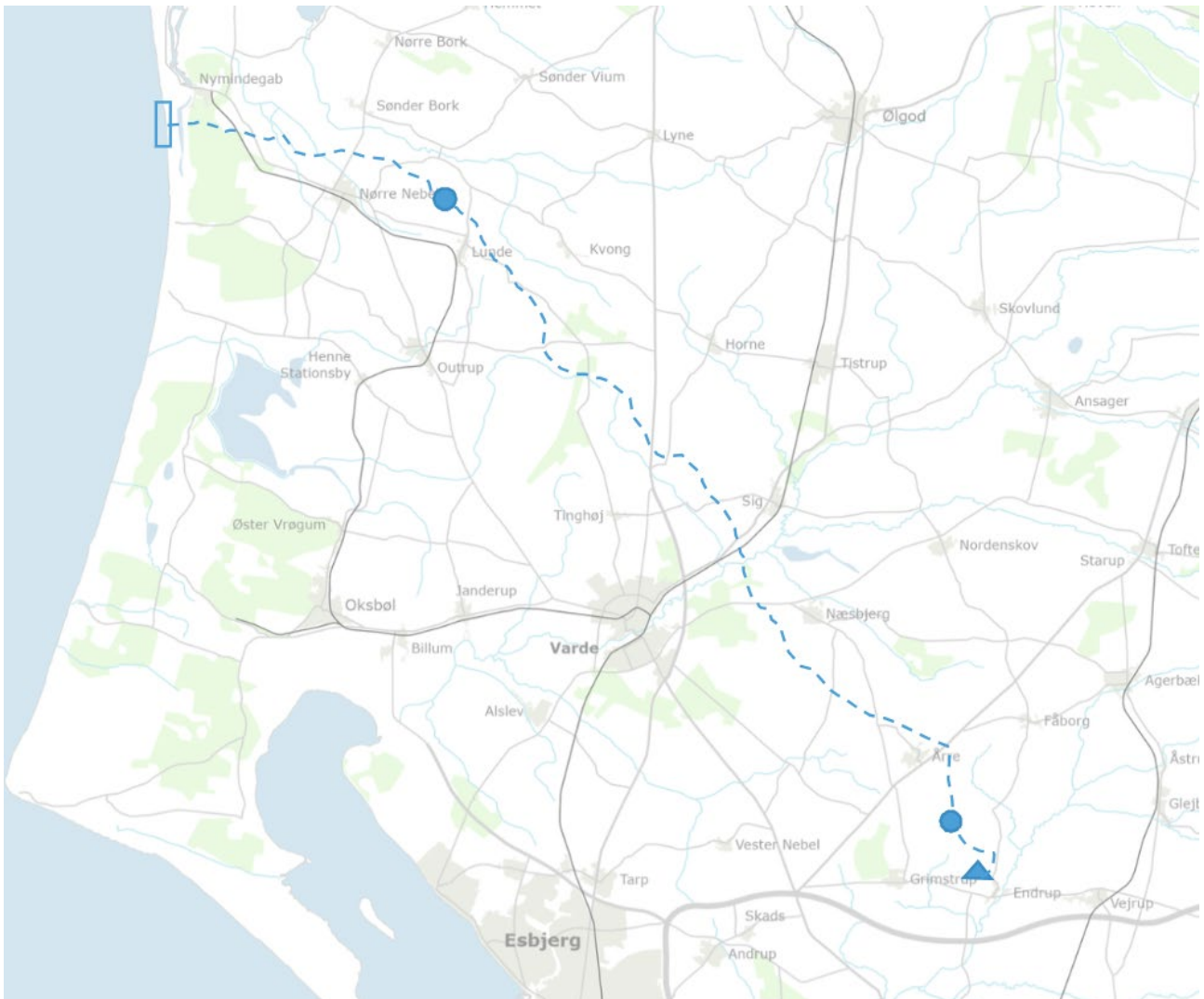
Figur 1- 1 Placering af projektet Mere Havvind 2030 Nordsøen I-A2 til Endrup, hvor firkanten angiver placering af ilandføringspunktet, cirklerne angiver placering af koncessionvinders anlæg (nord: kompensationsstation, syd: koblingsstation) og trekanten angiver placering af eksisterende højspændingsstation ved Endrup. Den stiplede linje angiver placering af landkabeltracé.
