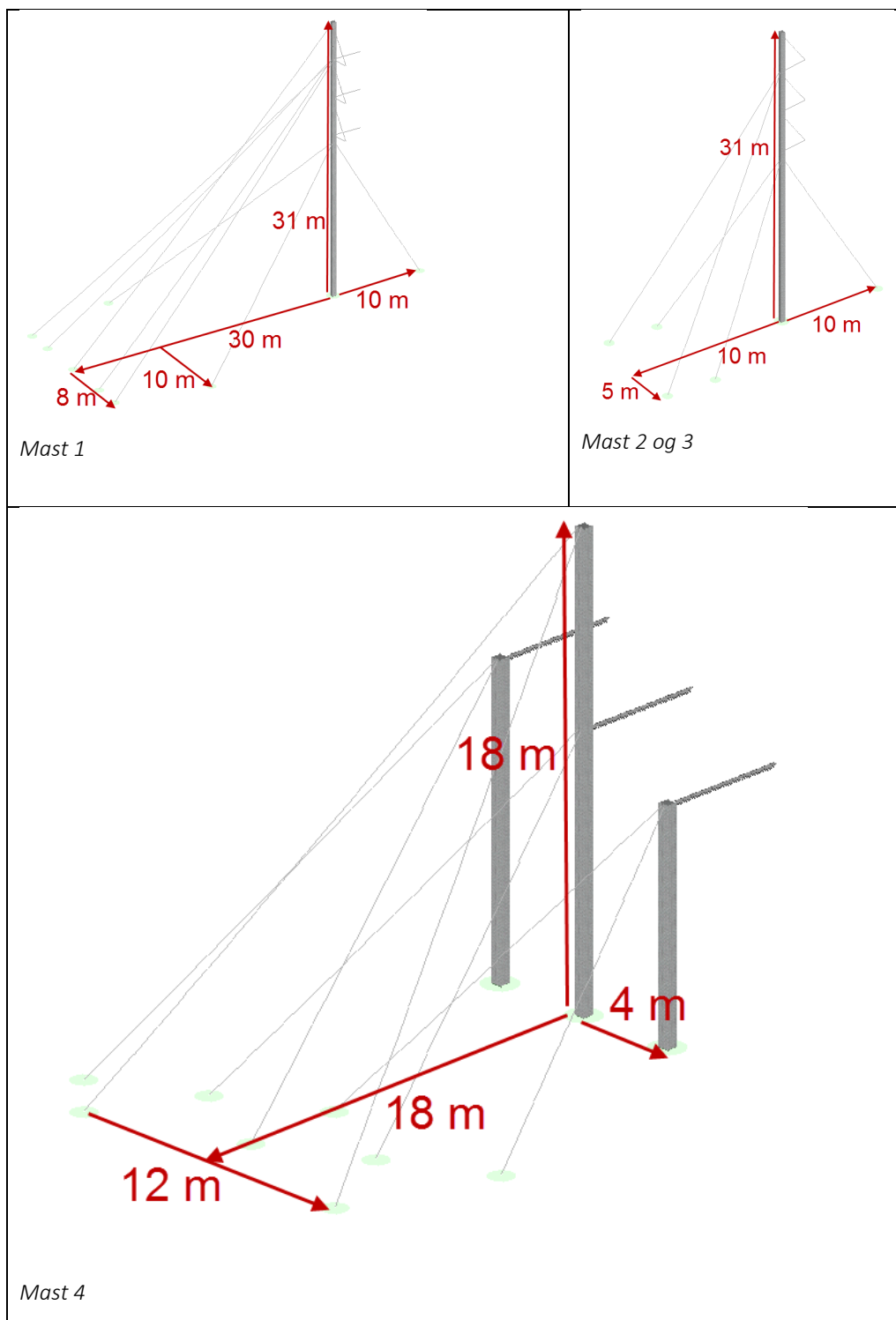
Figur 3. Oversigt over arealbehov for fastgørelse af barduner.
