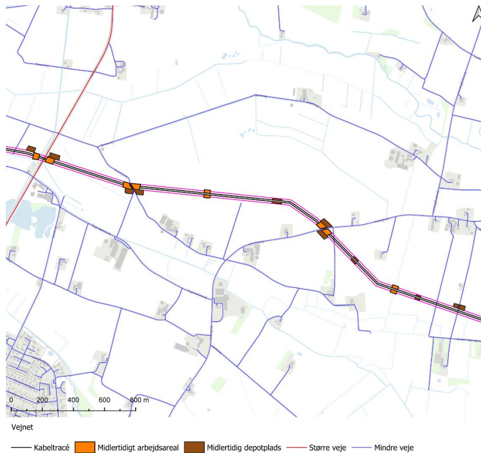
Figur 4: Kabeltracéets krydsning (fra vest mod øst) af Tarmvej (Rute 423) og Kvongvej
