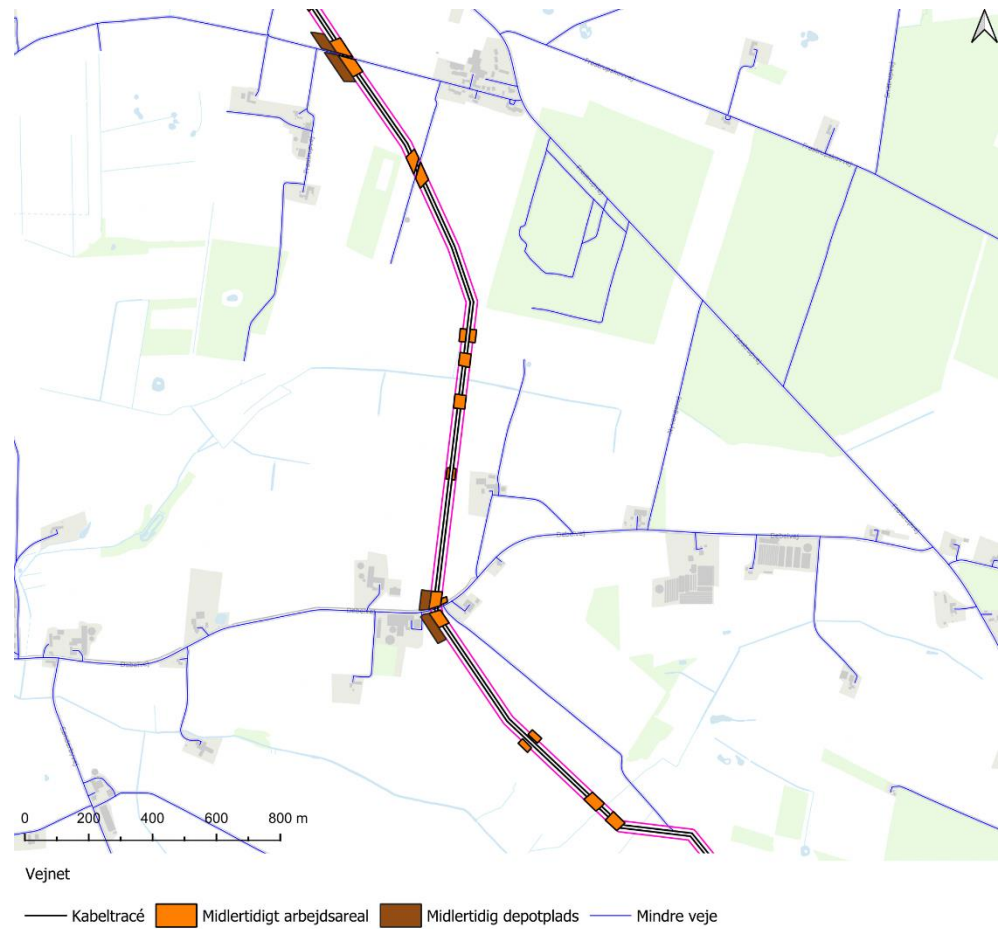
Figur 7: Kabeltracéets forløb forbi Frøstrup og Øster Debel med krydsning af Frøstrupvej og Debelvej
