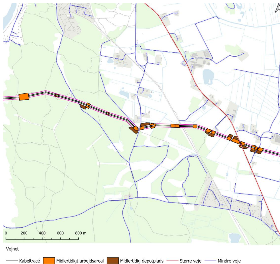
Figur 2: Kabeltracéets krydsning (fra vest mod øst) af Ulvedalvej, Søndre Klintvej, jernbanen og Vesterhavsvej (rute 181)
