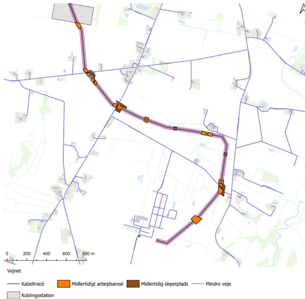
Figur 16: Kabeltracéets afsluttende forløb fra koblingsstationen med krydsning af Roustvej og Hjortkærvej
