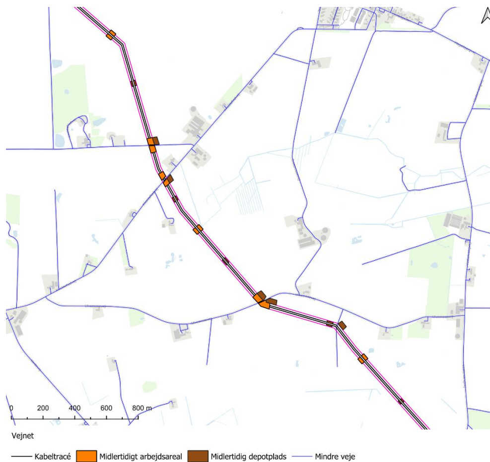
Figur 12: Kabeltracéets krydsning af Knoldeflodvej og Ulvemoosevej
