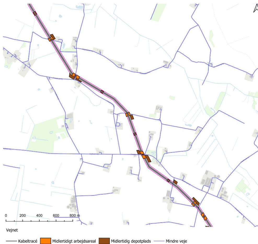
Figur 6: Kabeltracéets forløb forbi Skejdsbøl med krydsning af Skejdsbølvej og Frøstrupvej
