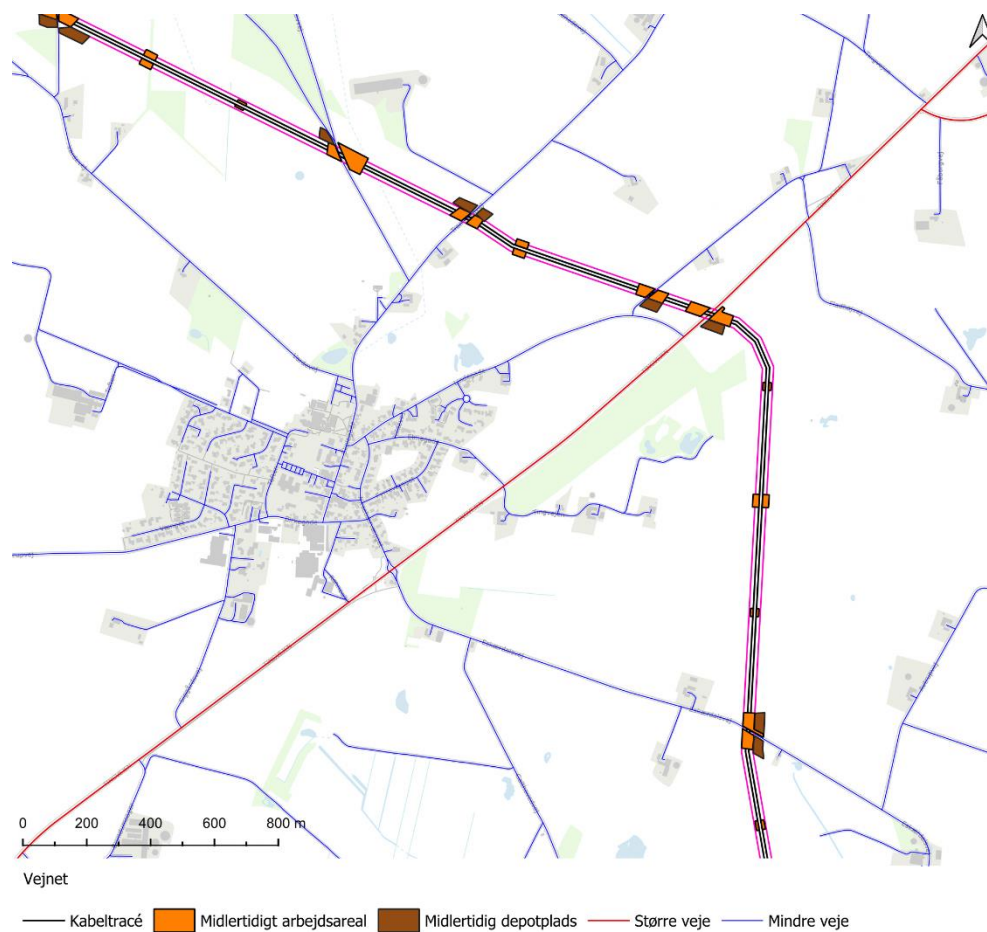
Figur 14: Kabeltracéets forløb nord om Årre og krydsning af Tingvejen (Rute 30)
