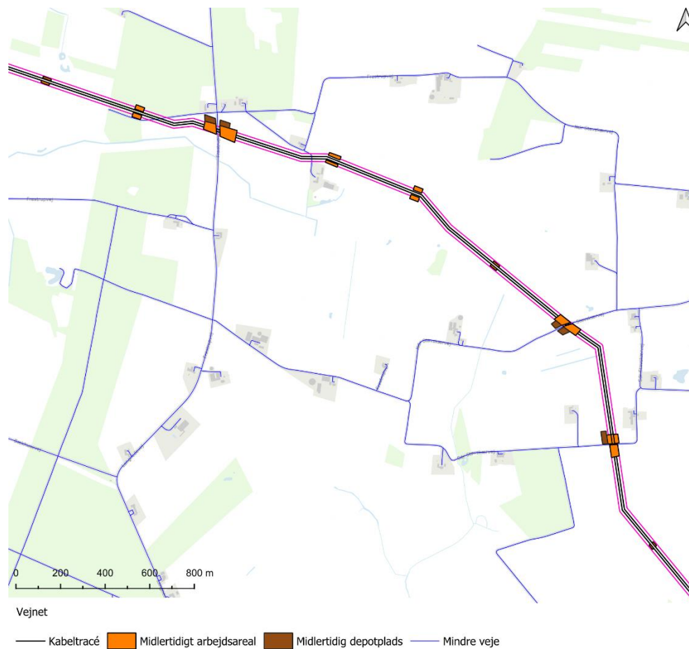
Figur 8: Kabeltracéets krydsning af Frøstrupvej nord for Søndersig samt Nordre og Søndre Stavskærvej
