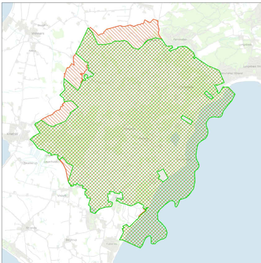
Figur 3. Habitatområde H186 Mols Bjerge med kystvande. Den røde skravering viser de berigtigede grænser for habitatområdet, og den grønne skravering angiver høringsforslagets afgrænsning. Dvs. at arealer, der kun er skraveret med grønt, er arealer, der er forslået tilføjet til det beskyttede område. Arealer, der kun er skraveret med rødt, er arealer, der er forslået fjernet fra det beskyttede område.
