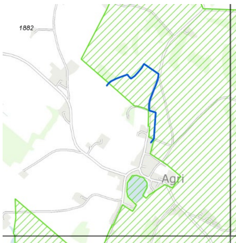
Figur 6. Tallene angiver nummeret på de kvadrater, hvis indhold behandles jf. figur 4. Den grønne skravering angiver høringsforslagets afgrænsning og den blå streg angiver den opdaterede områdegrense.
