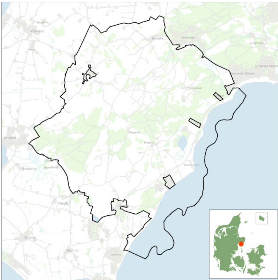
Figur 1. Gældende afgrænsning af Natura 2000-området N227 Mols Bjerge med kystvande.
