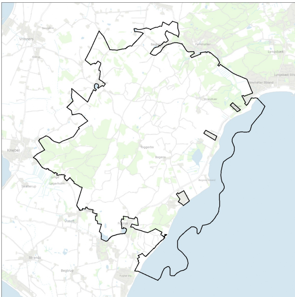
Figur 8. Den endelige afgrænsning af Natura 2000-område N227 fremgår af kortet.
