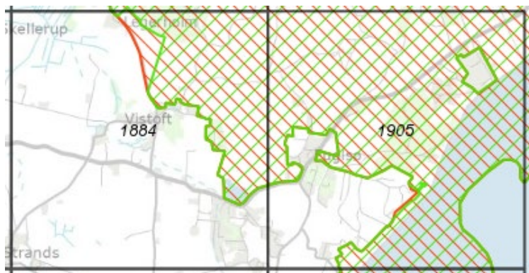
Figur 7. Tallene angiver nummeret på de kvadrater, hvis indhold behandles jf. figur 4. Den røde skravering viser de berigtigede grænser for habitatområdet, og den grønne skravering angiver høringsforslagets afgrænsning. Dvs. at arealer, der kun er skraveret med grønt, er arealer, der er forslået tilføjet til det beskyttede område. Arealer, der kun er skraveret med rødt, er arealer, der er forslået fjernet fra det beskyttede område.
