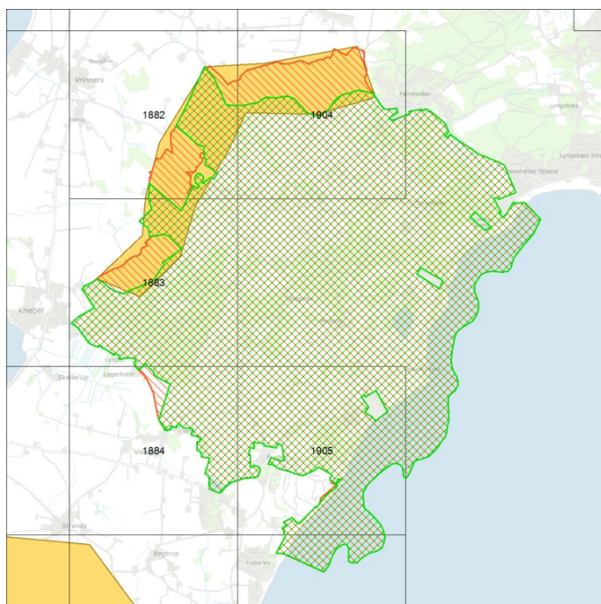
Figur 4. Habitatområde H182 Mols Bjerge med kystvande. Den røde skravering viser de berigtigede grænser for habitatområdet, og den grønne skravering angiver høringsforslagets afgrænsning. De gule og blå helfarvede polygoner viser ændringsforslagene, således at gul er forslag til udvidelse og blå er forslag til reduktion.
