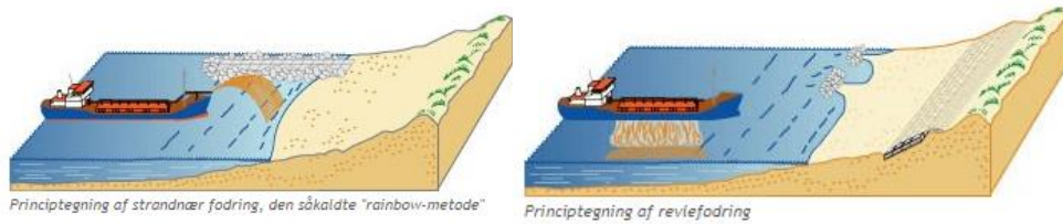
Figur 8-2. Kystfordringsmetoder fra havsiden: Kystnærfodring med enten 'rainrowing' (højre) eller splitting (venstre)
