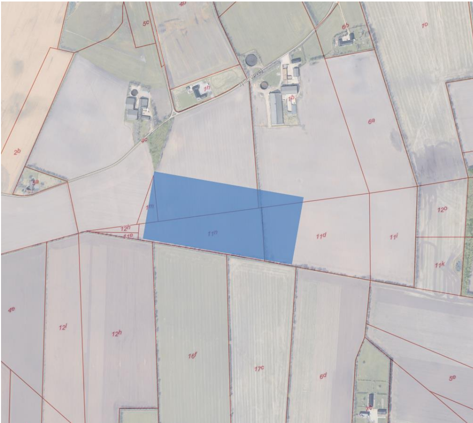
Figur 4-4. Den nye koblingsstation placeres i Vardø Kommune nord for den eksisterende station Endrup og tilkobles denne. Arealet til stationen udgør ca. 7,2 ha (400x180m).
