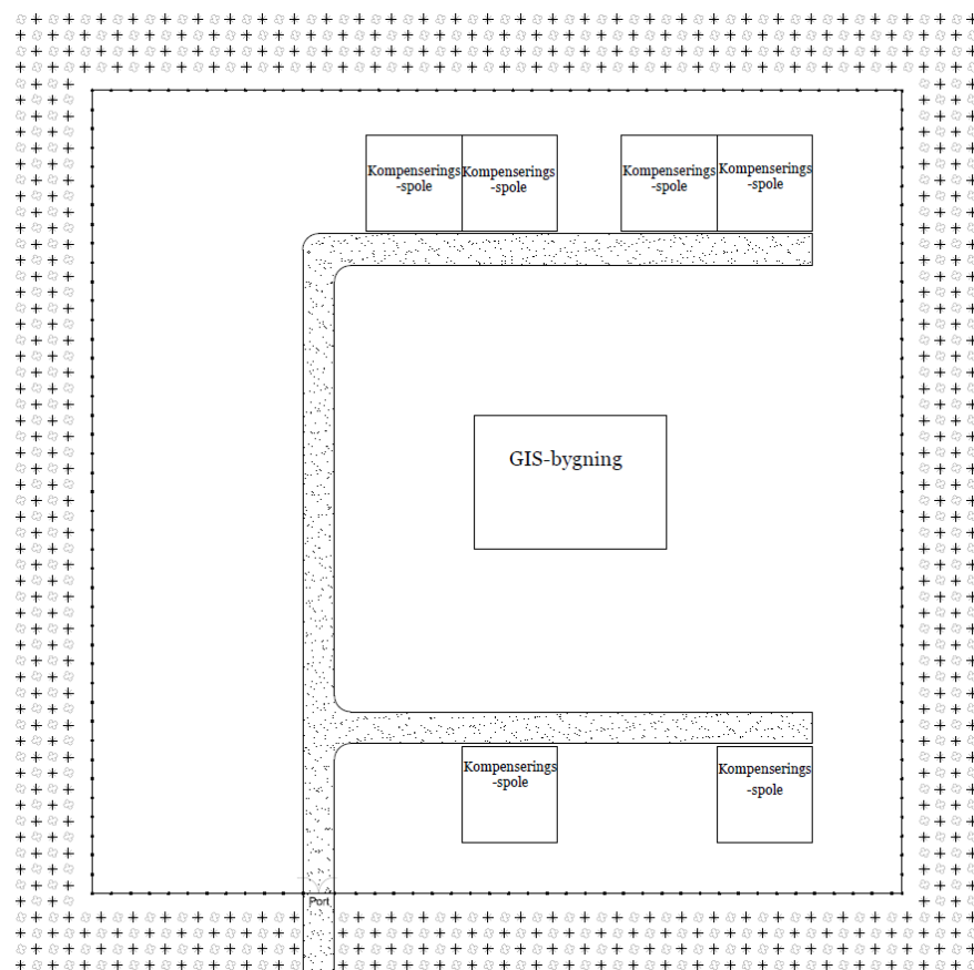
Figur 4-2 Eksempel på oversigtstegning over kompenseringsstation.
