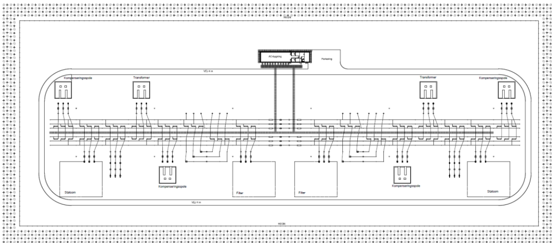
Figur 4-5 Oversigtstegning over koblingsstationen
