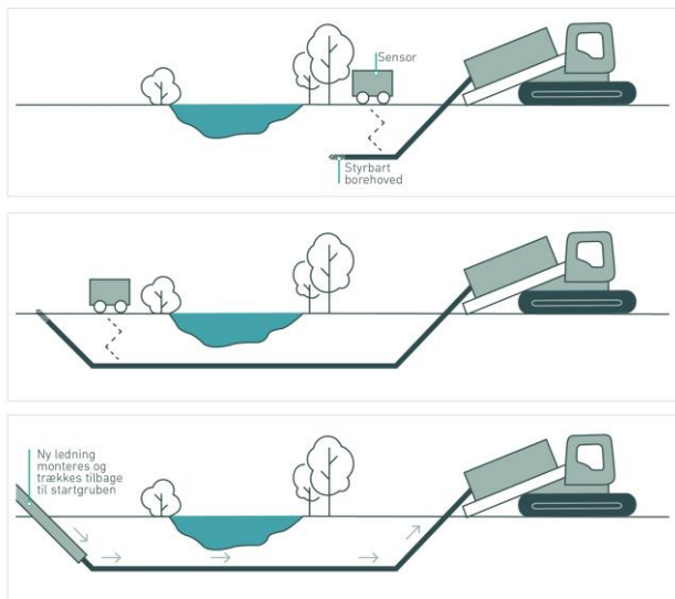
Figur 3-2: Arbejdsgangen ved styret underboring.
