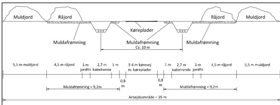
Figur 2-1 Princip for tværsnit af anlægsbælte til 275 kV kabelsystemer
