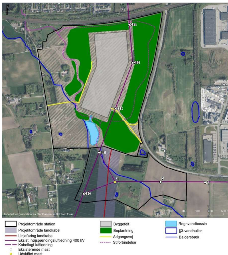
Figur 3. Fra ansøgningen. Indretning af stationsområde på Sjælland. De el-tekniske anlæg placeres i byggefeltet, som indhegnes.
